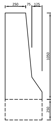
SECTION E - E
